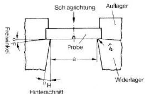
Bild 2: Widerlager und Auflager
