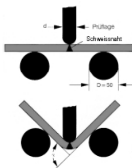
Bild 10: Biegeversuch
