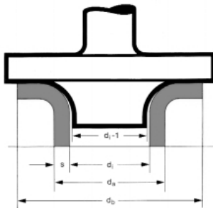
Bild 9: Bördelversuch
