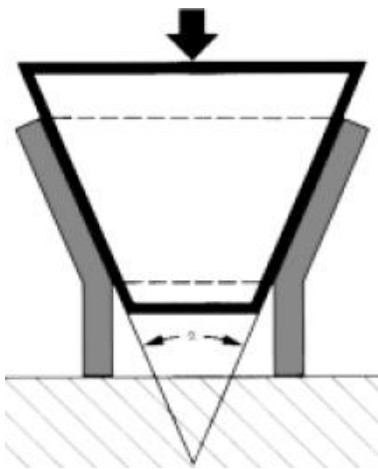
Bild 5: Aufweitversuch
