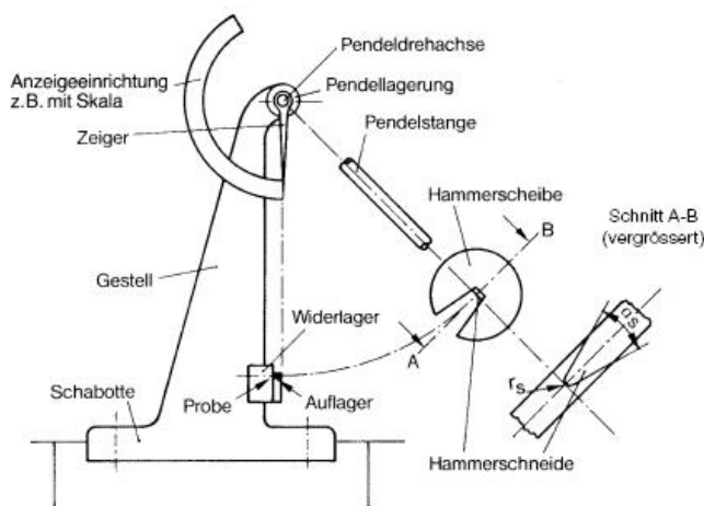
Bild 1: Pendelschlagwerk, schematisch
