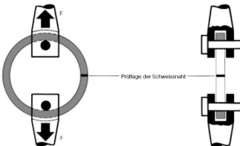
Bild 8: Ringzugversuch
